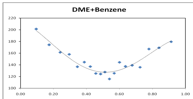
Fig. 4 DME + Benzene
