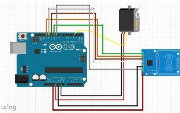
Fig.2.CircuitDiagramofRFIDTechnology
